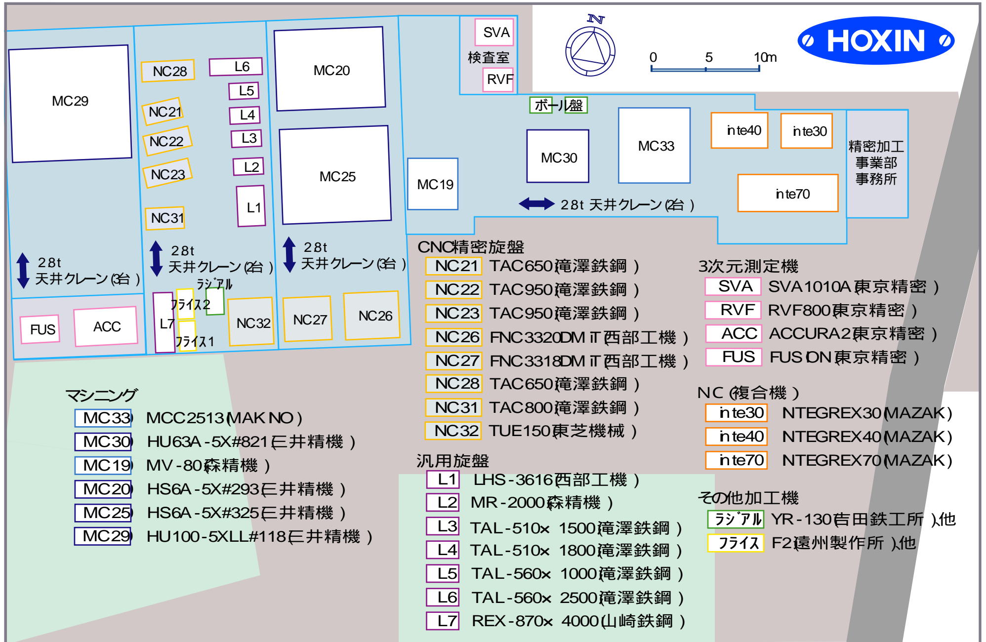
主要設備配置図
